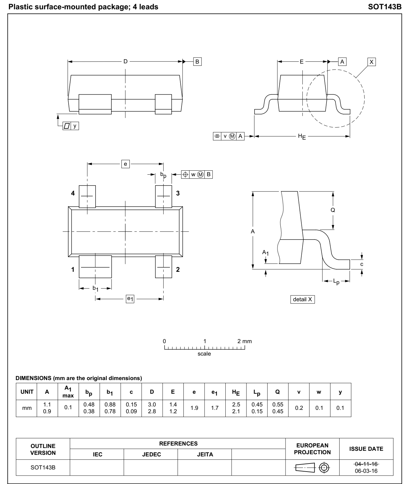
Fig 27. Package outline SOT143B
