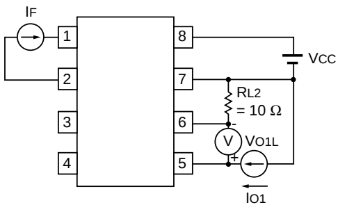
FIG. 1 ( V_{O1L} )
