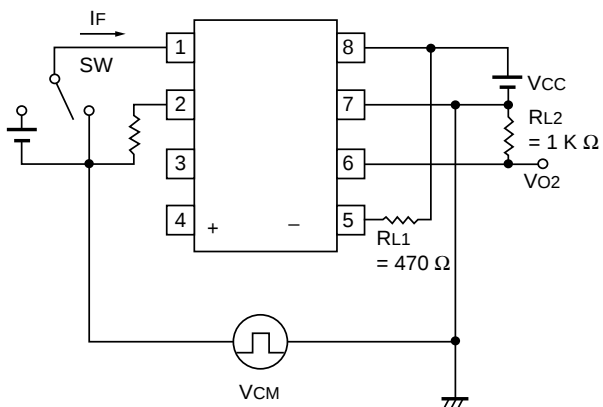
FIG. 7 ( CM_H , CM_L )
