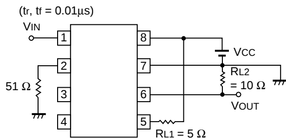
FIG. 6 ( t_{PLH} , t_{PHL} )
