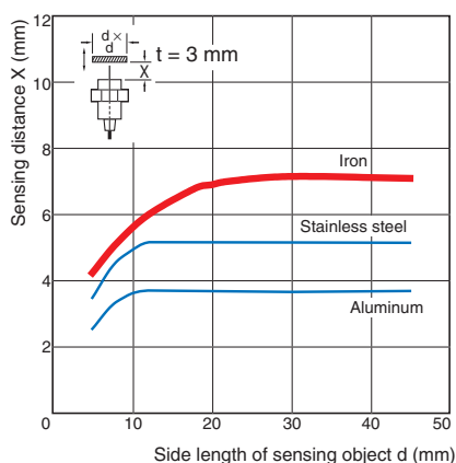
E2C-EM07M(-□)
