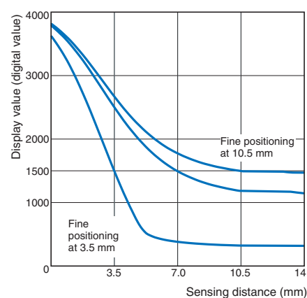
E2C-EM07M(-□)
