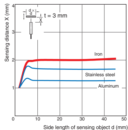
E2C-ED02(-□)/EM02(-□)
