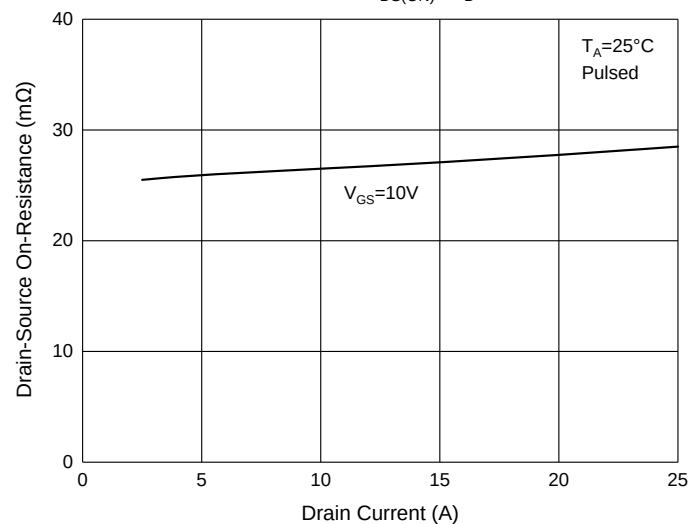
Fig. 6 - R_{DS(ON)} — I_D
