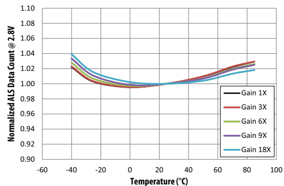
Figure 12 Normalized ALS Data Count @ 2.8V vs. Temperature
