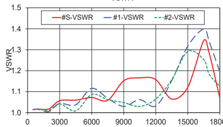
ZFRSC-183-S+ VSWR
