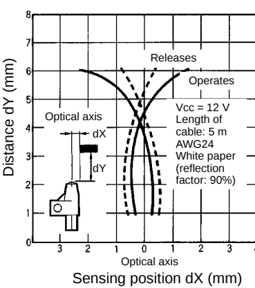
EE-SPZ301Y-01, EE-SPZ401Y-01
