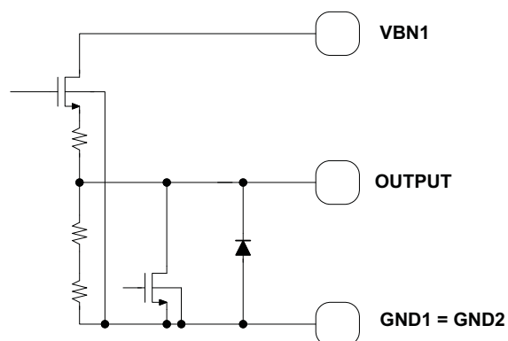
Figure 54. VREF1/VREF2
