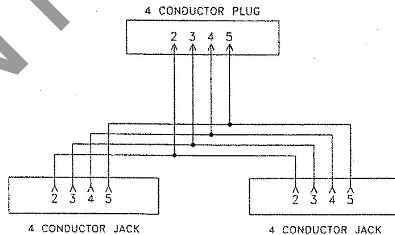
WIRING SCHEMATIC
